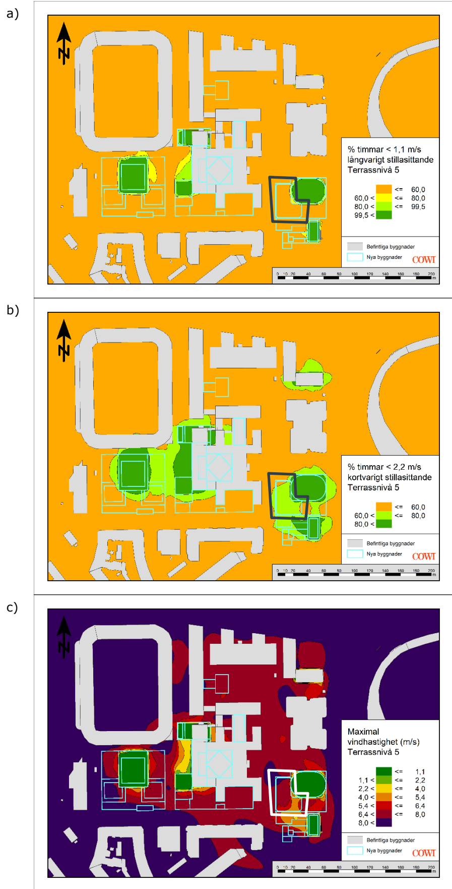
Figur 13. Vindkomfort på terrassnivå 5. Resultaten gäller för den markerade ytan.
